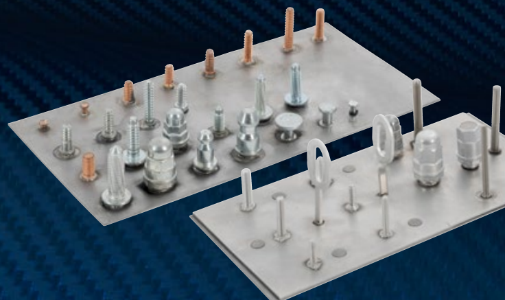
Stanznietenziehen
